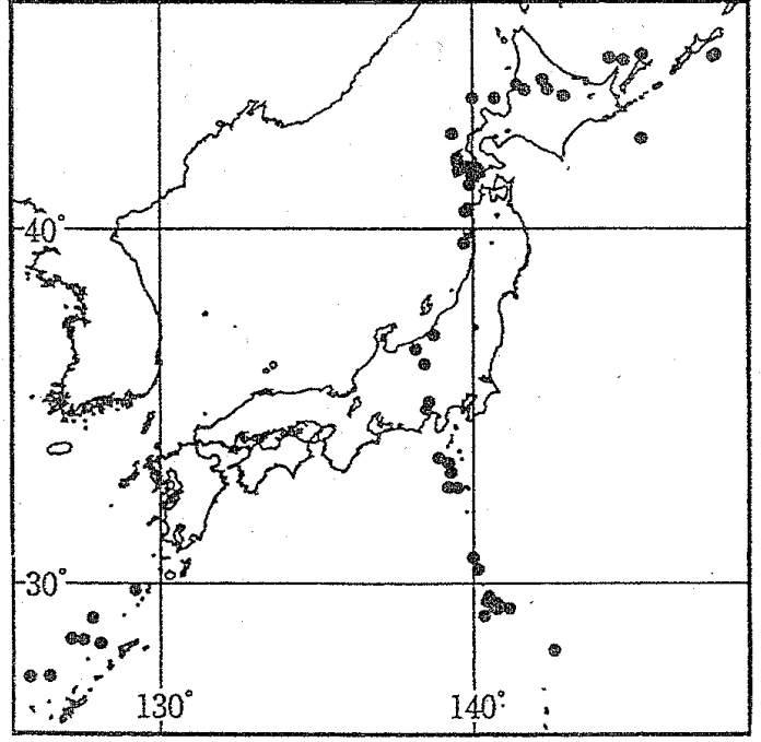
震源の深さ200km付近
