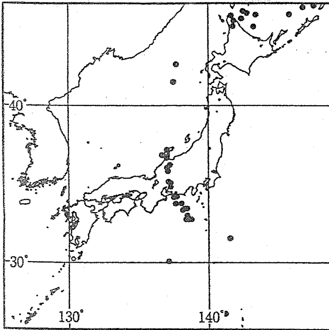
震源の深さ300km付近
