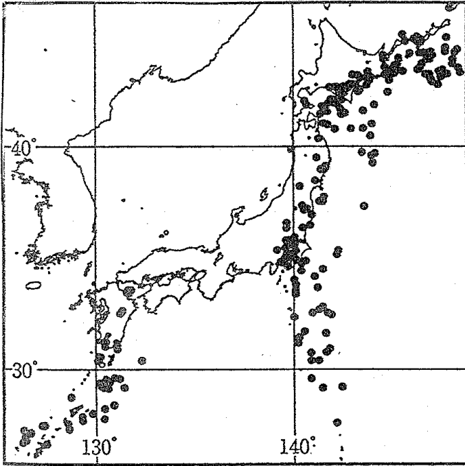
震源の深さ100km付近
