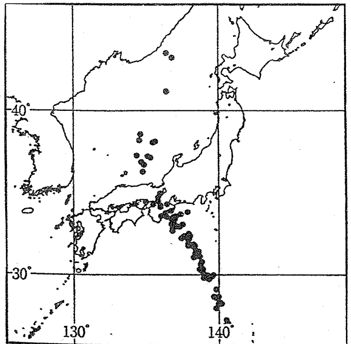
震源の深さ400km付近
